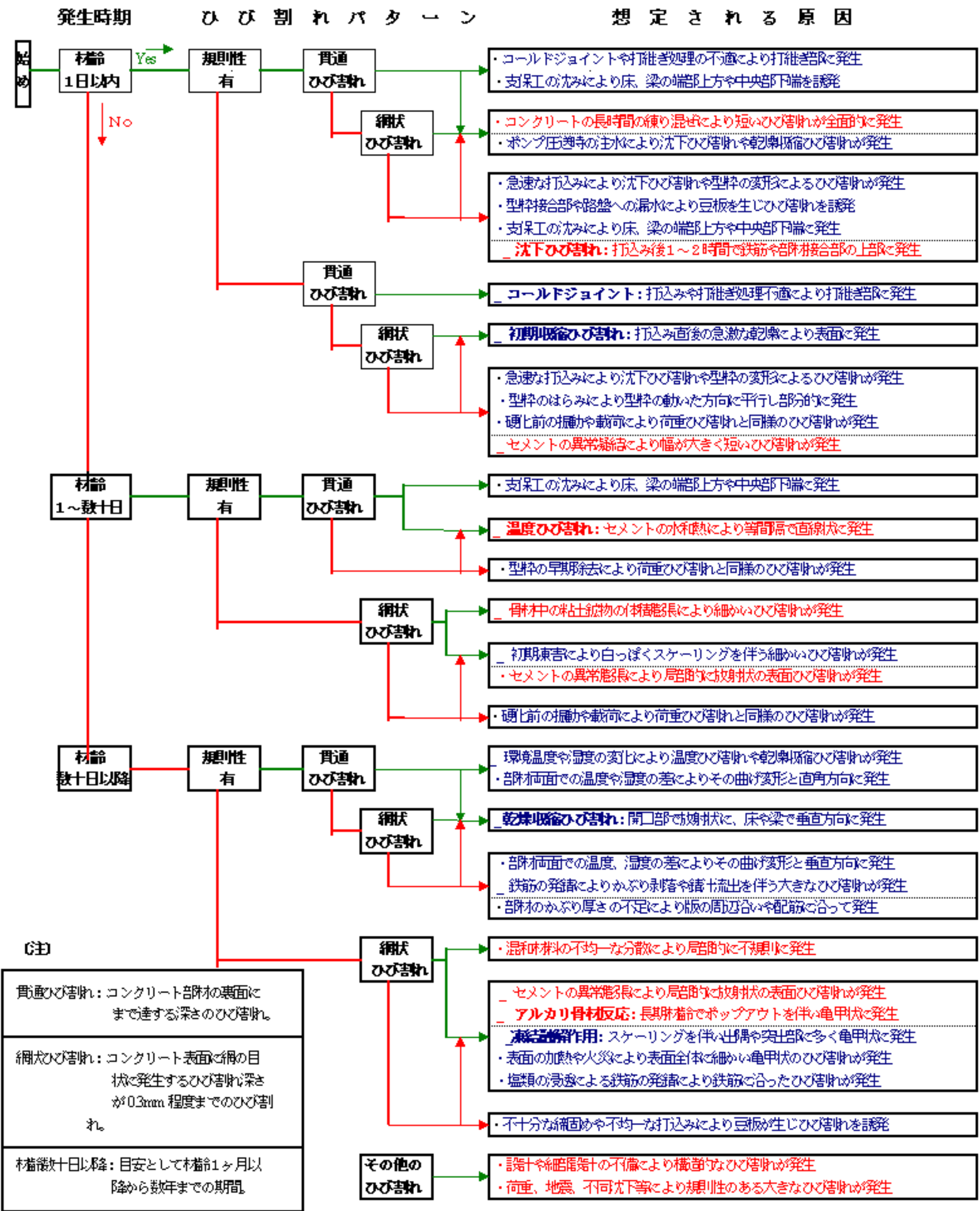
図1. ひび割れの発生時期およびパターンによる分類とその原因
